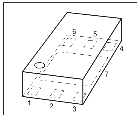
TSLP-7-4
