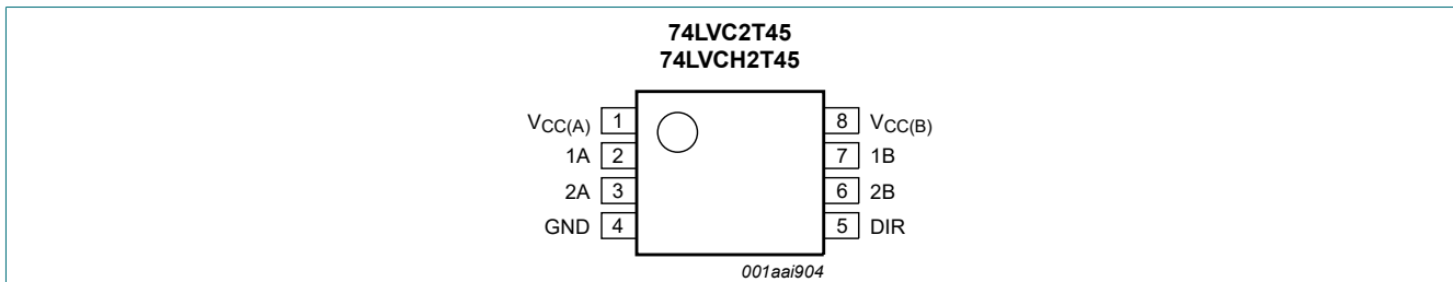
Fig. 3. Pin configuration SOT765-1 (VSSOP8)
