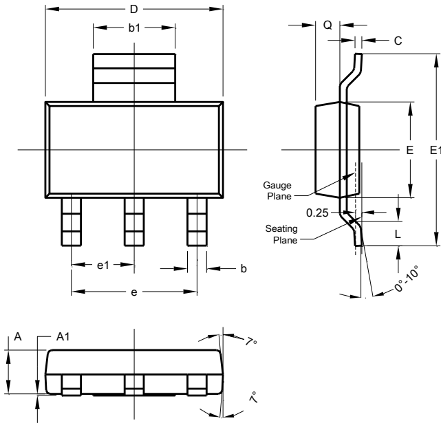
SOT223
