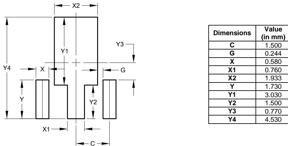
SOT89
