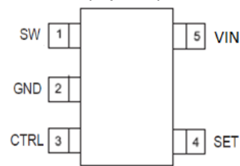
TSOT25
