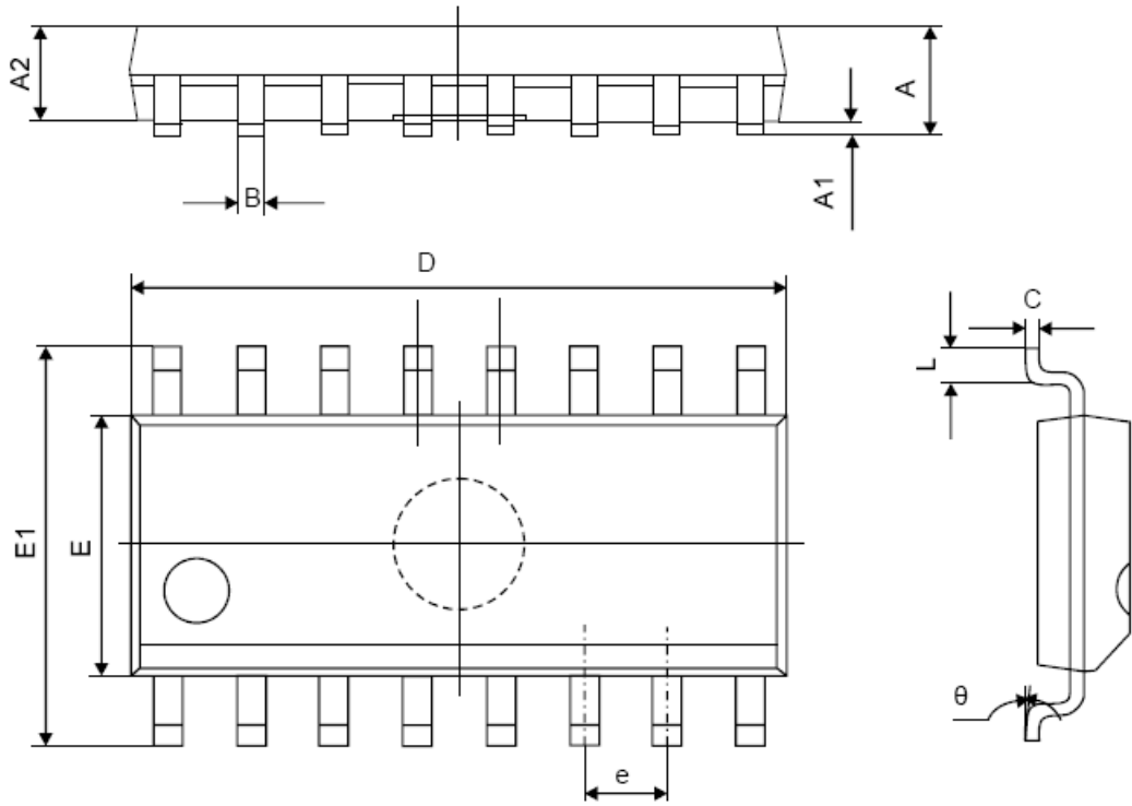
SOP-16
