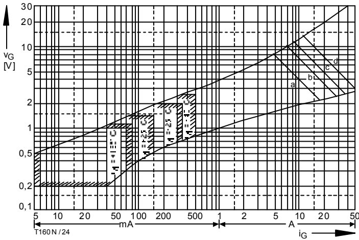
Bild / Fig. 24 Steuercharakteristik mit Zündbereichen / Gate characteristic with triggering areas V_G = f(i_G) , V_D = 6 V
