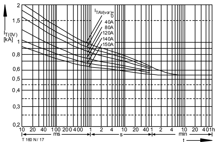
Bild / Fig. 15 Überstrom / Overload on-state current I_{T(OV)} = f(t) Verstärkte Luftkühlung / Forced air-cooling, t_A = 35 \text{ °C} Kühlkörper / Heatsink: K0.55-M12-A, V_L = 50 \text{ l/s} Parameter: Vorlaststrom / Pre-load current I_{TAV(vor)}
