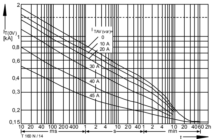
Bild / Fig. 14 Überstrom / Overload on-state current I_{T(OV)} = f(t) Luftselbstkühlung / Natural air-cooling, t_A = 45 \text{ °C} Kühlkörper / Heatsink: K0.11-M12-A Parameter: Vorlaststrom / Pre-load current I_{TAV(vor)}
