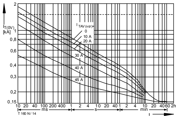
Bild / Fig. 15 Überstrom / Overload on-state current I_{T(OV)} = f(t) Verstärkte Luftkühlung / Forced air-cooling, t_A = 35 \text{ °C} Kühlkörper / Heatsink: K0.11-M12-A, V_L = 30 \text{ l/s} Parameter: Vorlaststrom / Pre-load current I_{TAV(vor)}
