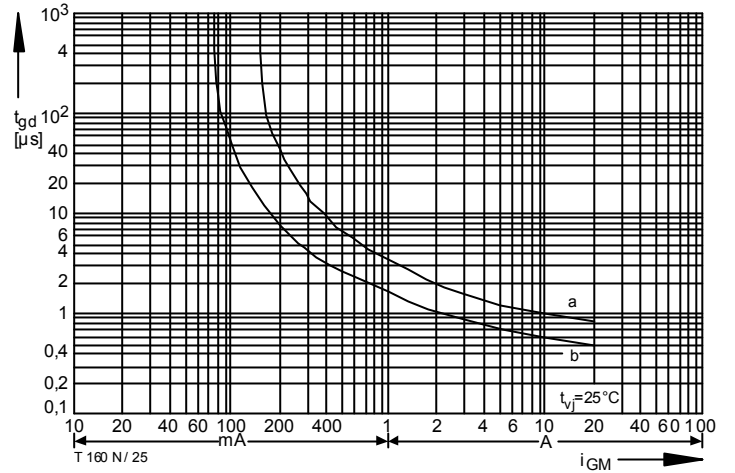
Bild / Fig. 25 Zündverzögerung / Gate controlled delay time t_{gd} = f(i_{GM}) t_{vj} = 25^\circ\text{C} , di_G/dt = i_{GM}/1\mu\text{s}
