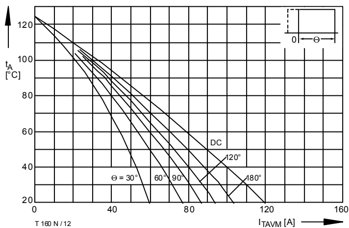
Bild / Fig. 12 Höchstzulässige Kühlmitteltemperatur / Max. allowable cooling medium temperature t_A = f(I_{TAVM}) Luftselbstkühlung / Natural air-cooling Kühlkörper / Heatsink: K0.55-M12-A Parameter: Stromflußwinkel / Current conduction angle \theta
