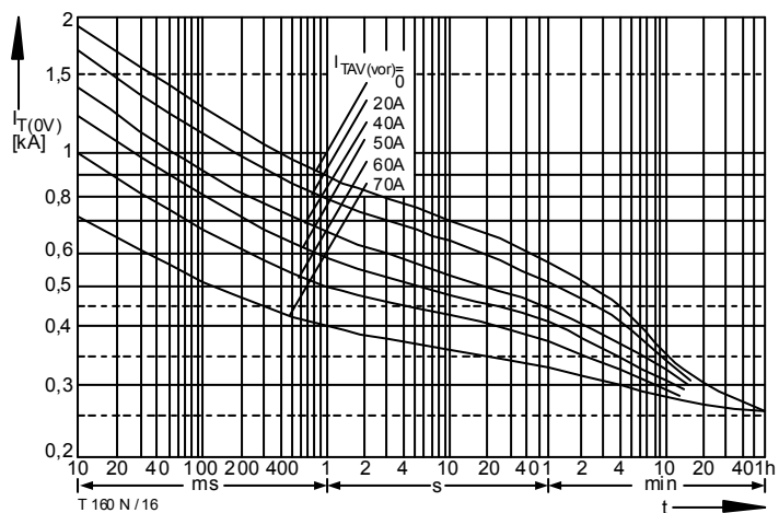
Bild / Fig. 16 Überstrom / Overload on-state current I_{T(OV)} = f(t) Luftselbstkühlung / Natural air-cooling, t_A = 45 \text{ °C} Kühlkörper / Heatsink: K0.55-M12-A Parameter: Vorlaststrom / Pre-load current I_{TAV(vor)}
