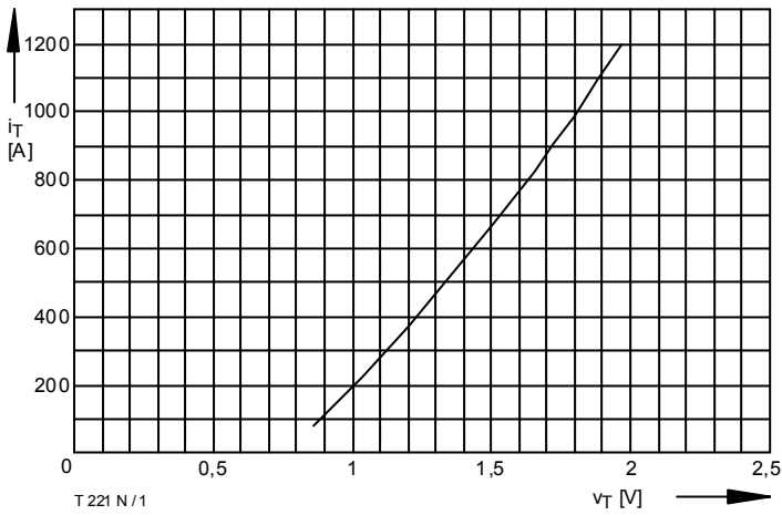
Bild / Fig. 1 Durchlaßkennlinie / On-state characteristic i_T = f(v_T) , t_{vj} = t_{vj \text{ max}}
