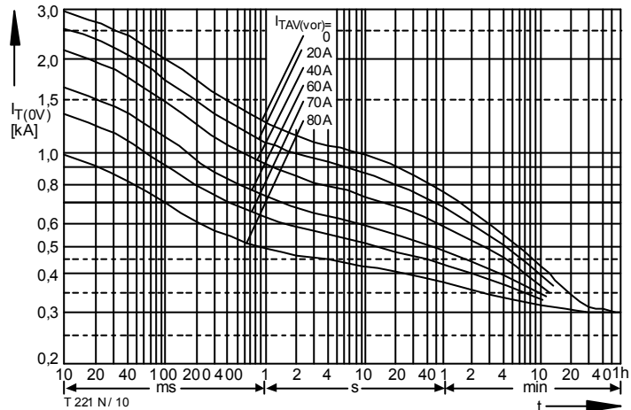
Bild / Fig. 10 Überstrom / Overload on-state current I_{T(OV)} = f(t) Luftselbstkühlung / Natural air-cooling, t_A = 45 °C Kühlkörper / Heatsink: K0.55-FB54-A Parameter: Vorlaststrom / Pre-load current I_{TAV(vor)}
