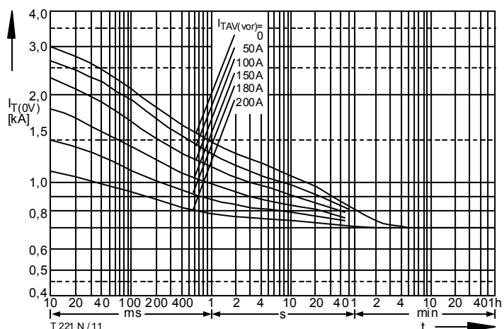
Bild / Fig. 11 Überstrom / Overload on-state current I_{T(OV)} = f(t) Verstärkte Luftkühlung / Forced air-cooling, t_A = 35 °C Kühlkörper / Heatsink: K0.55-FB54-A, V_L = 50 l/s Parameter: Vorlaststrom / Pre-load current I_{TAV(vor)}
