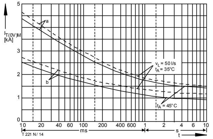
Bild / Fig. 14 Grenzstrom / Max. overload on-state current I_{T(OV)M} = f(t) , V_{RM} = 0,8 V_{RRM} - - - - - Luftseltkühlung / Natural air-cooling, t_A = 45^\circ\text{C} - - - - - Verstärkte Luftkühlung / Forced air-cooling, t_A = 35^\circ\text{C} Kühlkörper / Heatsink: K0.55-FB54-A, V_L = 50\text{ l/s} Belastung aus / Surge current occurs: a - Leerlauf / No-load conditions b - Betrieb mit Dauergrenzstrom / During operation at max. average on-state current I_{TAVM}
