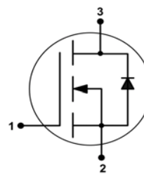
PG-SOT23
