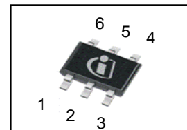
PG-SOT363
