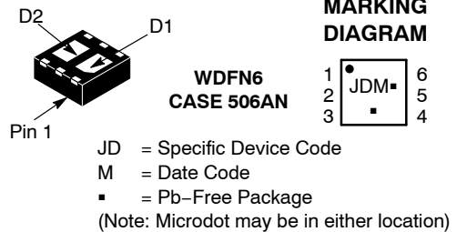
P-CHANNEL MOSFET P-CHANNEL MOSFET
