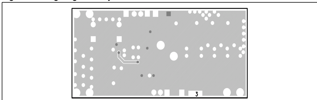
Figure 25. Bottom layer
