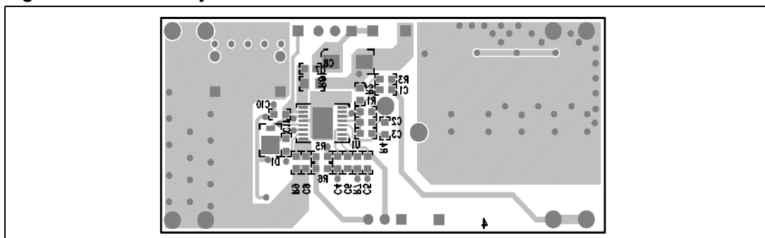
Figure 25. Bottom layer
