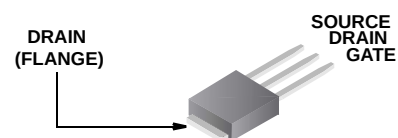
JEDEC TO-251AA
