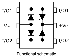
SOT23-6L
