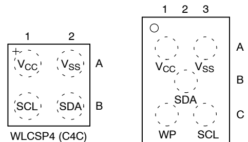
WLCSP4 (C4C)
