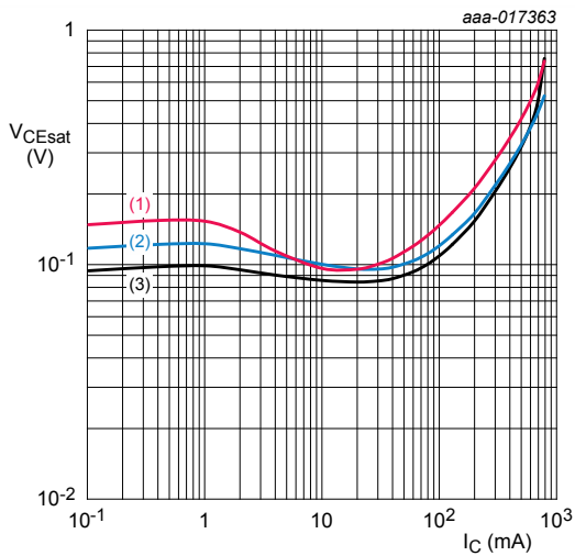
I_C/I_B = 20 (1) T_{amb} = 150 °C (2) T_{amb} = 25 °C (3) T_{amb} = -55 °C
