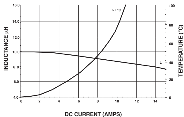
IHLP-5050CE-01 10 \mu H
