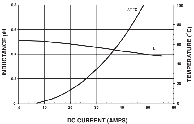
IHLP-5050CE-01 0.47 \mu H
