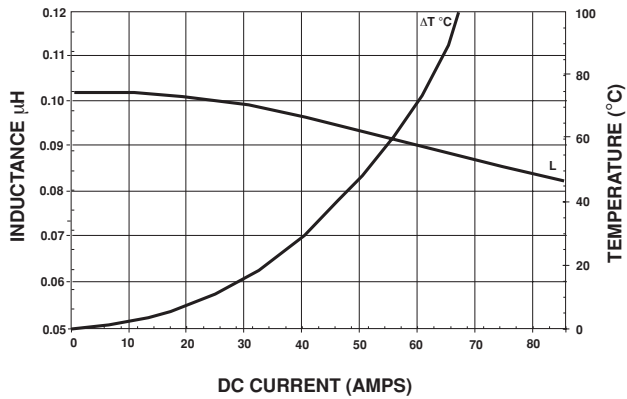
IHLP-5050CE-01 0.10 \mu H
