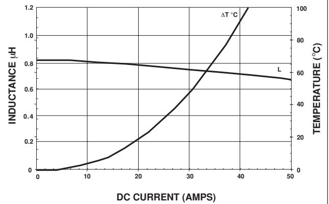
IHLP-5050CE-01 0.82 \mu H
