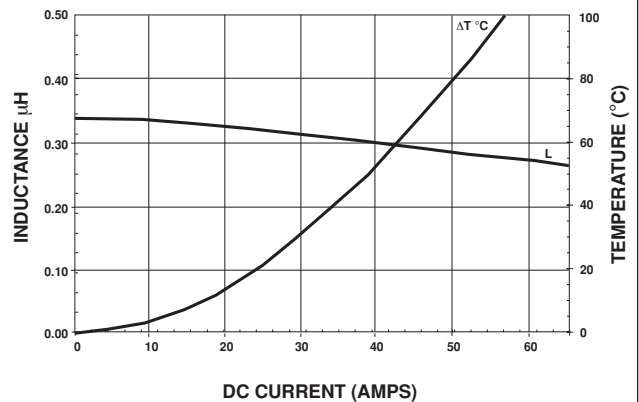
IHLP-5050CE-01 0.33 \mu H
