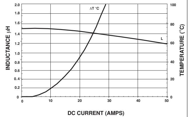
IHLP-5050CE-01 1.5 \mu H
