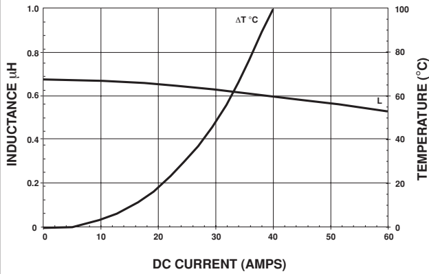
IHLP-5050CE-01 0.68 \mu H
