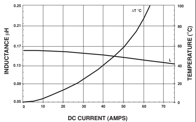
IHLP-5050CE-01 0.15 \mu H
