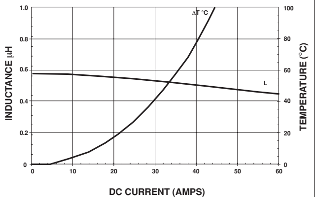
IHLP-5050CE-01 0.60 \mu H
