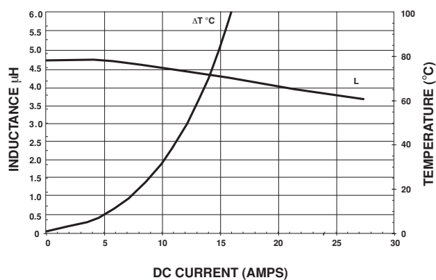
IHLP-5050CE-01 4.7 \mu H
