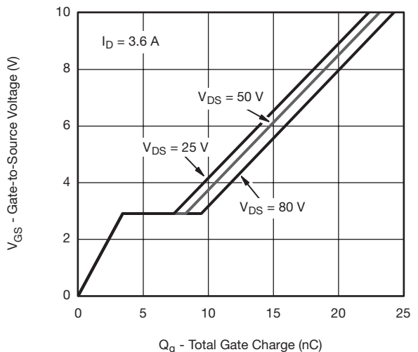
I_D = 3.6 A V_{DS} = 50 V V_{DS} = 25 V V_{DS} = 80 V Gate Charge
