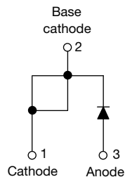
TO-220AC
