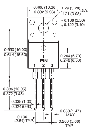
ITO-220AB
