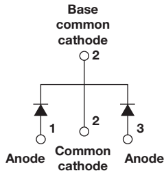
TO-263AB (D 2 PAK)
