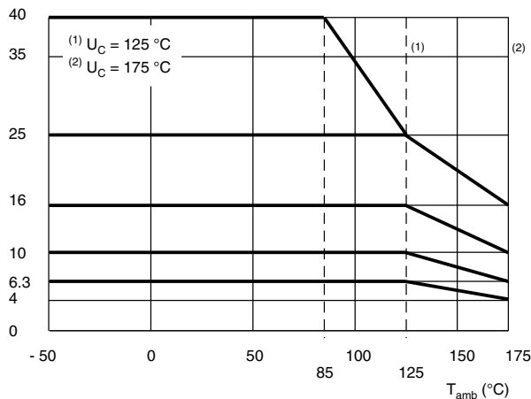
Fig. 5 - Maximum permissible voltage up to T amb = 175 °C
