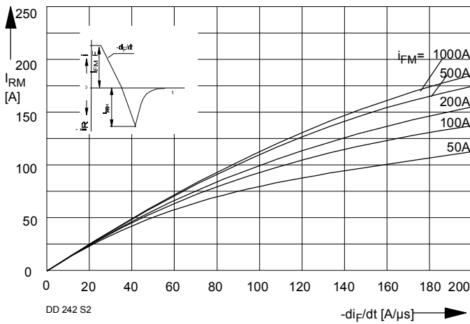
Bild / Fig. 1 Typische Abhängigkeit der oberen Rückstromspitze von der abkommütierenden Stromsteilheit -di_F/dt bei t_{vj \max} . Typical relationship between the maximum peak reverse current and the rate of decay of forward current -di_F/dt at t_{vj \max}
