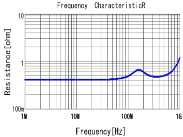
■ DE11XRA150KN4AQ01F R DCOV, 20degC
