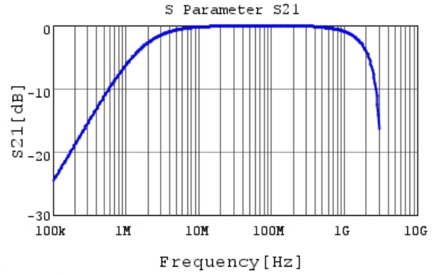
DE2E3KY102MB3BU02F S21 DCOV, 20degC
