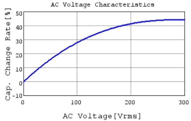
DE2E3KY102MB3BU02F C-AC Voltage capchange, I
