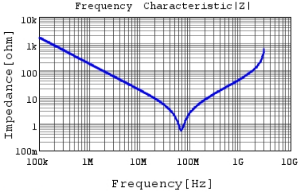
DE2E3KY102MB3BU02F |Z| DC0V, 20degC
