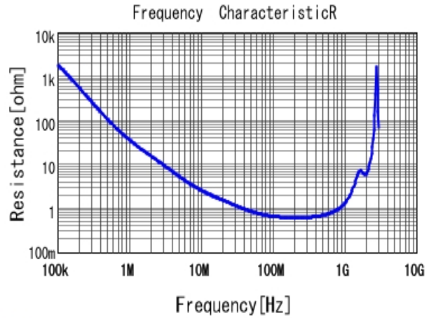
■ DE2B3KY151KB2BM01F R DCOV, 20degC
