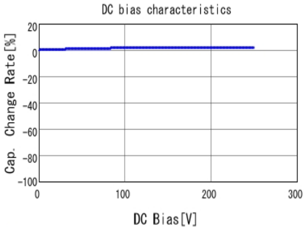
■ DE2B3KY221KN3AM02F C-DC bias capchange, 20.0degC, AC1
