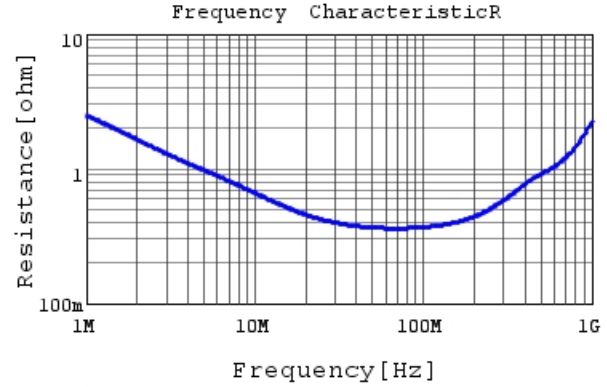
DE2E3SA222MN3AX02F R DCOV, 20degC
