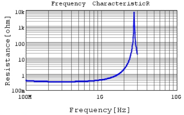
DE21XKY220JA2BM01F R DCOV, 20degC
