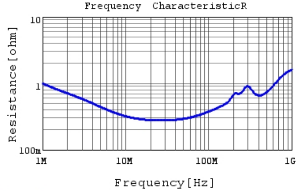
DE2E3SA472MA3BX02F R DC0V, 20degC
