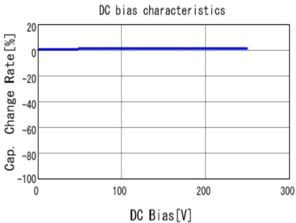
■ DE2B3KY331KN3AM02F C-DC bias capchange, 20.0degC, AC1
