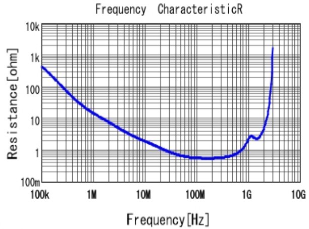
■ DE2B3KY331KN3AM02F R DCOV, 20degC
