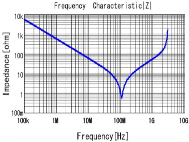
■ DE2B3KY331KN3AM02F |Z| DCOV, 20degC
