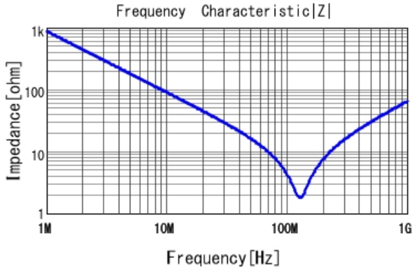
DE2B3SA221KA2BT01F |Z| DCOV, 20degC
