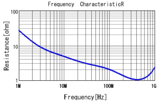
DE2B3SA221KA2BT01F R DCOV, 20degC
