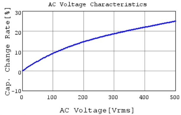
DE1B3RA471KA4BQ01F C-AC Voltage capchange, I
