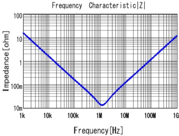
■ ECASD41E106M040KA0 |Z| DCOV, 25degC
