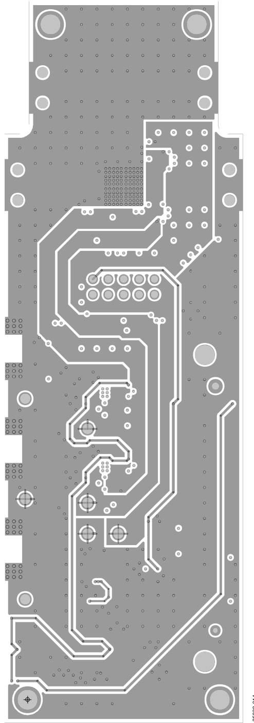
Figure 14. ADMV8818-EVALZ Layer 3
