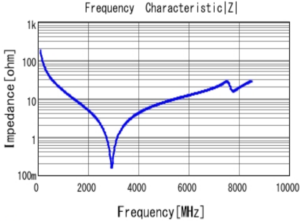
■ GCQ1555C1H8R8CB01 |Z| DC0V, 25degC
