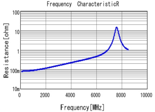
■ GCQ1555C1H8R8CB01 R DC0V, 25degC
