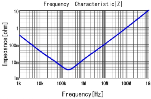
■ ECASD60E477M4R5K00 |Z| DC0V, 25degC
