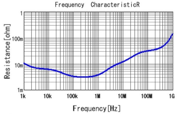
■ ECASD60E477M4R5K00 R DC0V, 25degC
