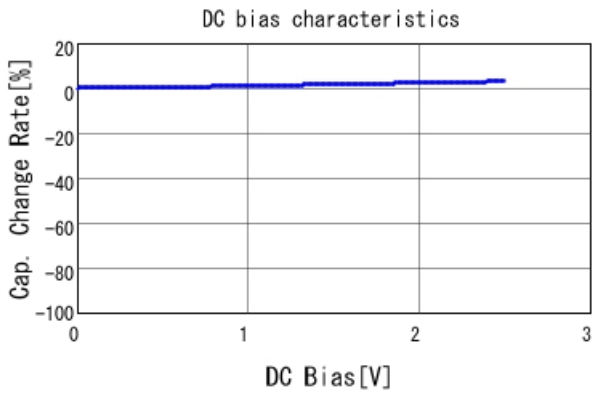
■ ECASD60E477M4R5K00 C-DC bias capchange, 25.0degC, AC1
