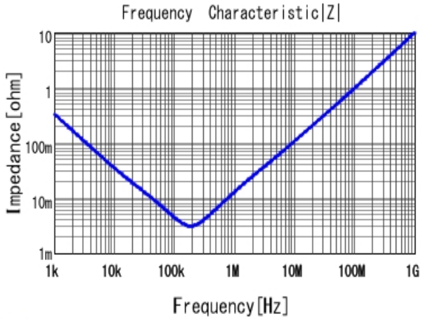
■ ECASD60E477M006K00 |Z| DCOV, 25degC
