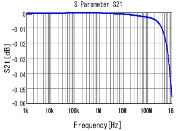
■ ECASD60E477M006K00 S21 DCOV, 25degC
