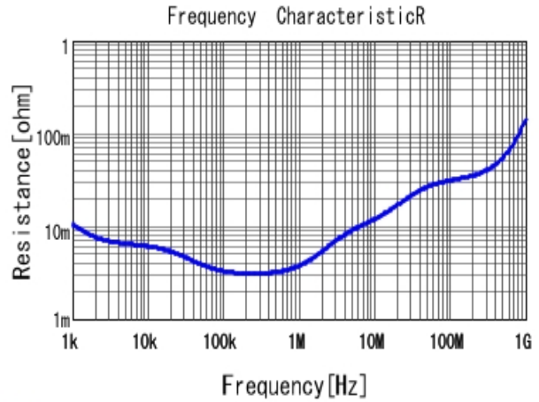
■ ECASD60E477M006K00 R DCOV, 25degC
