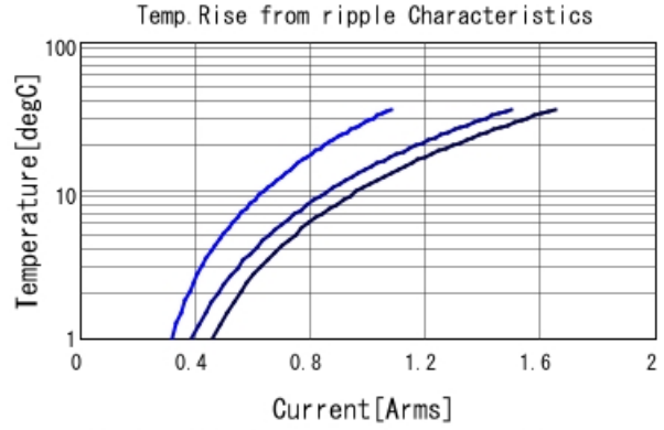
GRM188R71E104KA01 Temp. rise — 400kHz — 800I
