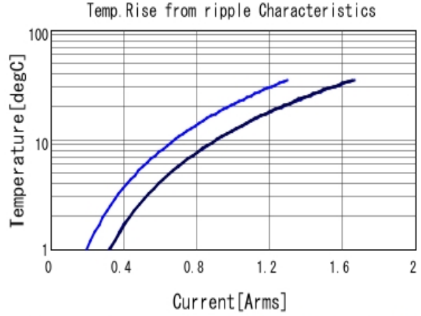
GRM188R72A104KA35 Temp. rise ■ 400kHz ■ 800kHz ■ 1MHz
