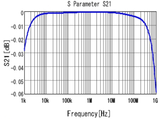
■ ECASD41E226M040KA0 S21 DCOV, 25degC
