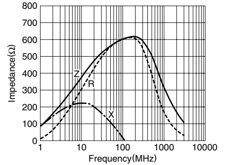
MMZ1608R601C
