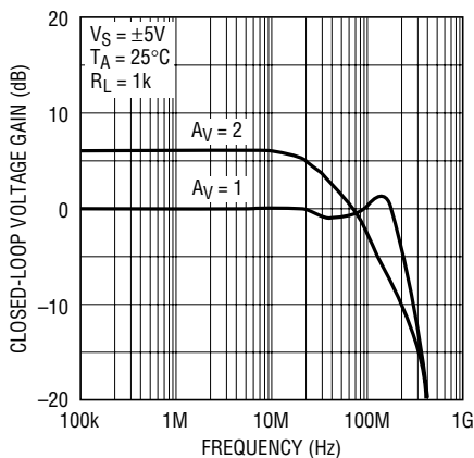
LT1190 • TA05
