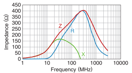
MPZ1608S331ATD25
