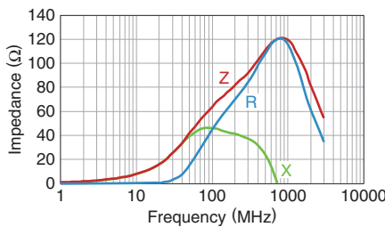
MPZ1608Y600BTD25
