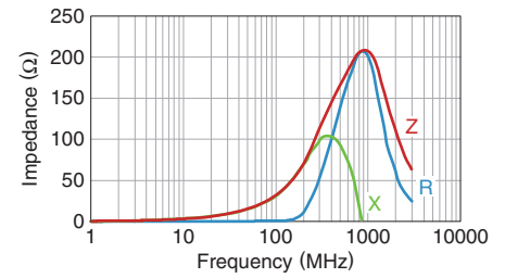
MPZ1608D300BTD25
