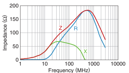
MPZ1608S121ATDH5
