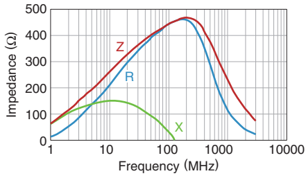
MPZ1608B471ATD25
