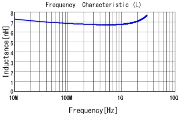
LQW15AN6N8H0Z L
