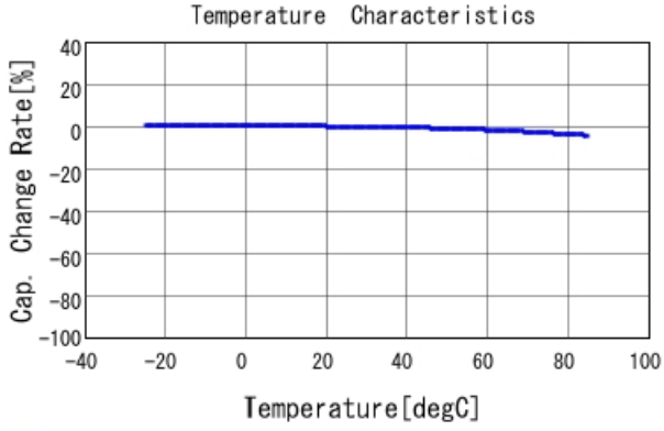
■ GRM033B31H152KA12 C-Temp. capchange, DCO. 0V, AC1. 0Vrm
