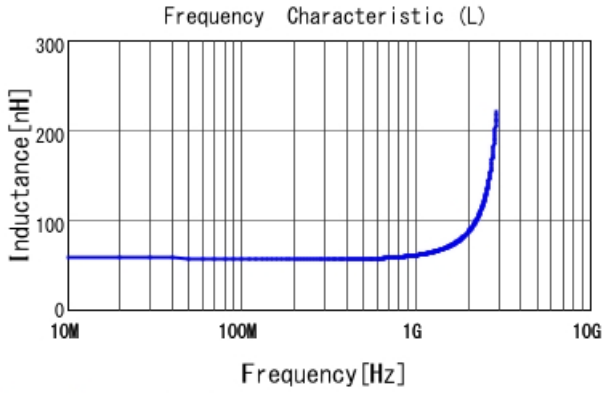
LQW15AN56NH0Z L
