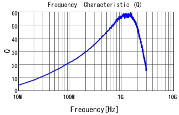
LQW15AN56NH0Z Q
