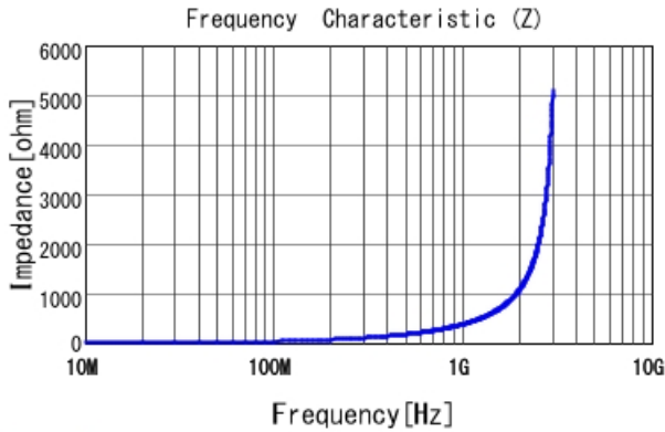
LQW15AN56NH0Z |Z|
