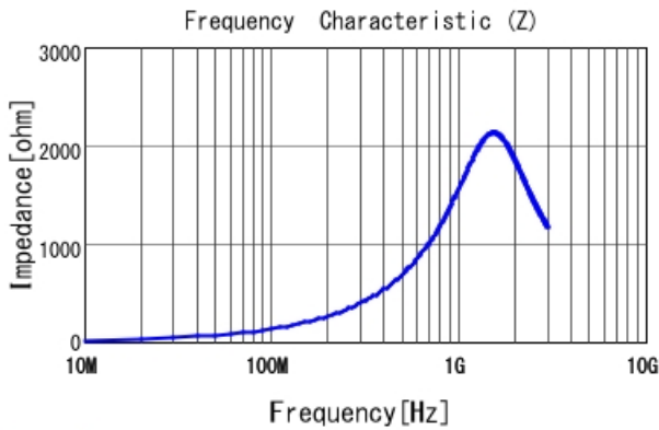
LQW15CAR22K00 |Z|
