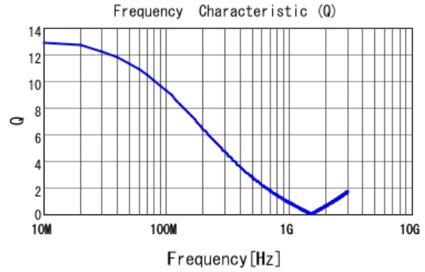
LQW15CAR22K00 Q
