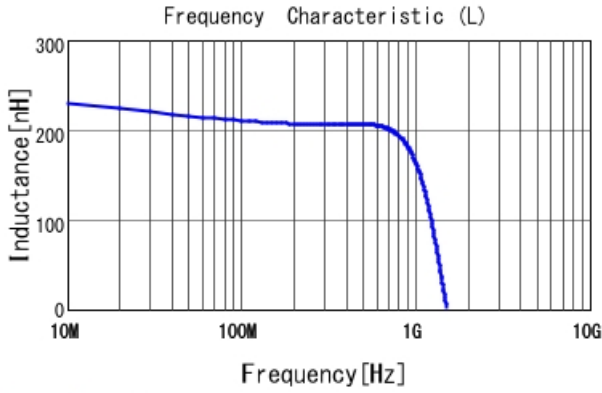
LQW15CAR22K00 L
