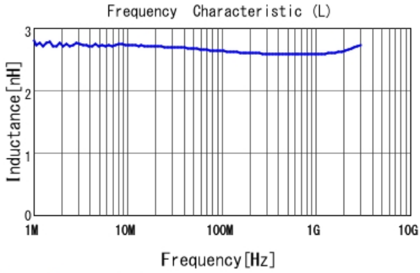
LQW15AN2N7G80 L
