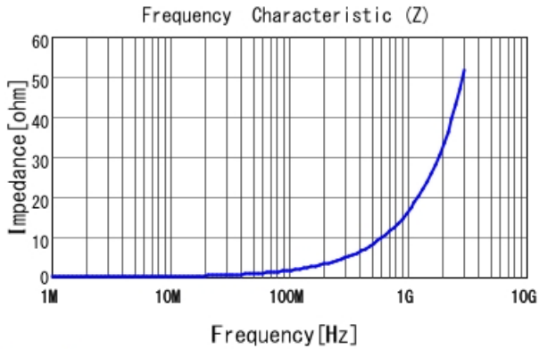
LQW15AN2N7G80 |Z|
