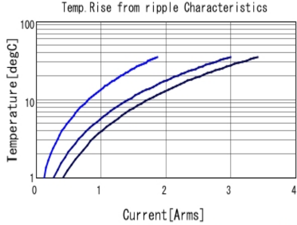
GRM316B31C225KA87 Temp. rise ■ 100kHz ■ 500kHz ■ 1MHz
